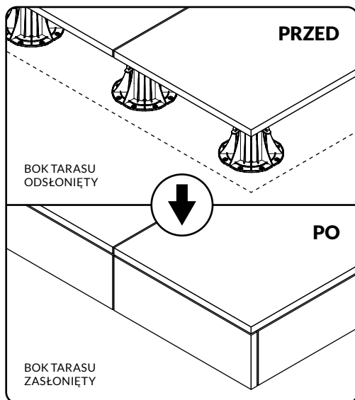
Zestaw montażowy do maskownic tarasu na wspornikach - element podstawowy
